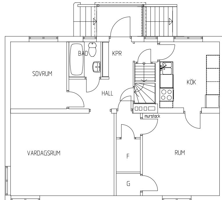
ENTRÉPLAN 1:100
